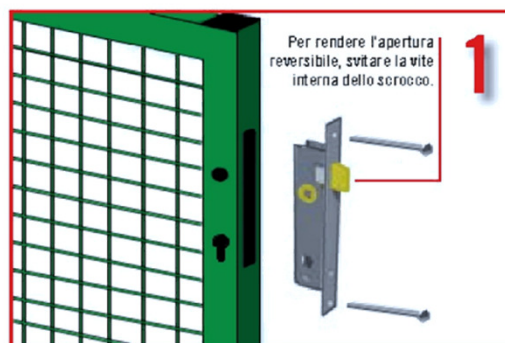
1 - Inserire la serratura nell'apposito alloggiamento
